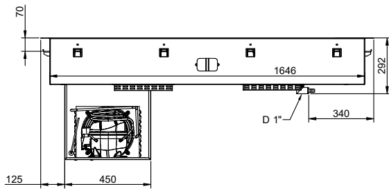
Côté
