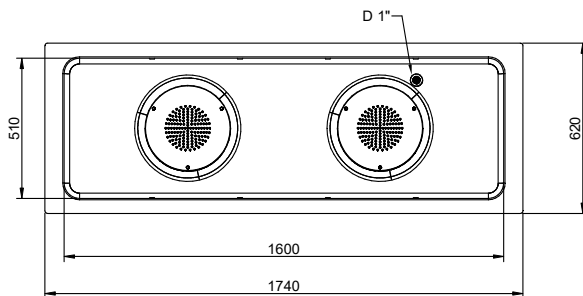
Dessus
